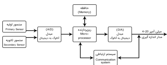
شکل ۳ بخش های یک ترانسمیتر خبره با یک مرکز ارتباطی [۳]
