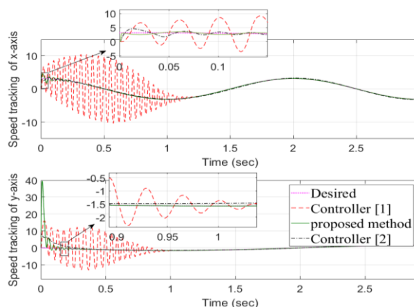
شکل ۶: تحول زمانی ردیابی سرعت
