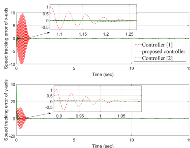
شکل ۷: تحول زمانی خطاهای ردیابی سرعت
