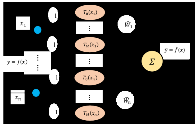
شکل ۱: ساختار شبکه عصبی چپیشف
