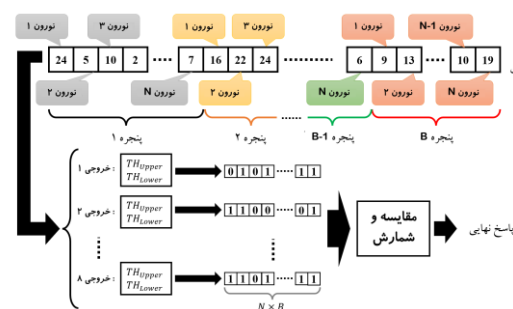
شکل ۵: فرآیند تبدیل نرخ آتشی متوالی به بردار صفر و یک و تشخیص
