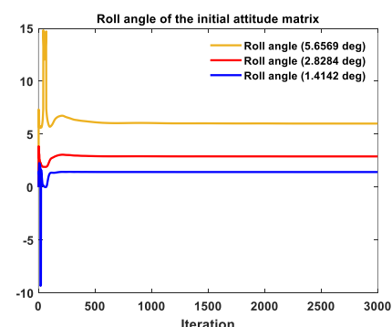
شکل ۵: نمایش از تخمین زاویه غلت در ماتریس وضعیت اولیه در شرایط ترازیابی در حین حرکت
