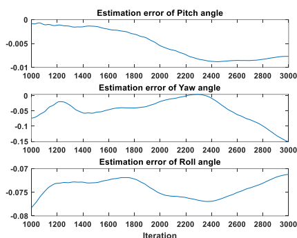
شکل ۷: نمایی از خطای وضعیت در ترازیابی با روش انتگرال‌گیری از
