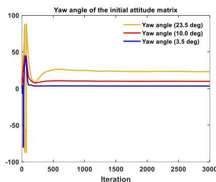
شکل ۴: نمایش از تخمین زاویه سمت در ماتریس وضعیت اولیه در شرایط ترازیابی در حین حرکت
