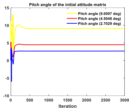
شکل ۸: نمایی از تخمین زاویه فراز در ماتریس وضعیت اولیه در شرایط
