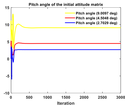
شکل ۸: نمایشی از تخمین زاویه فراز در ماتریس وضعیت اولیه در شرایط
