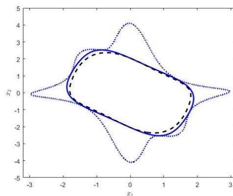
شکل ۶: منحنی سیاه خط چین تخمین ناحیه جذب بر اساس فیدبک حالت [۲۲]، منحنی آبی خط پیوسته تخمین DA با روش پیشنهادی، منحنی آبی نقطه چین
