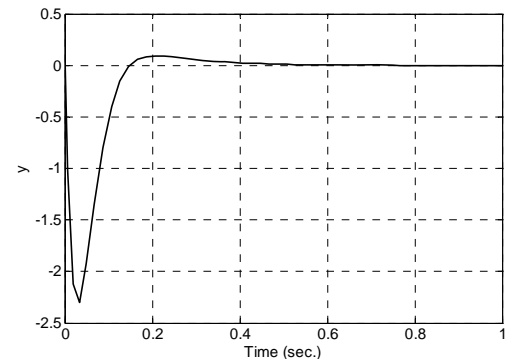
شکل ۸: خروجی سامانه با بازخورد خروجی پویای مرتبه دو برای هر زیر سامانه
