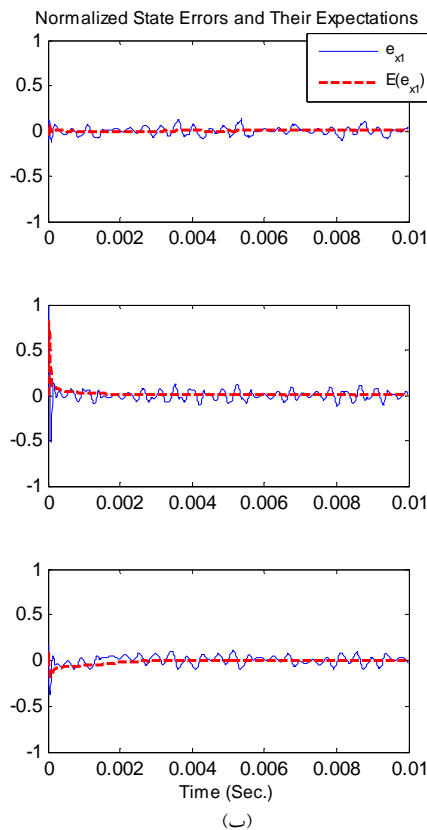
شکل (۱): (الف) حالت‌های راه‌انداز (آبی، خط توپر) و پاسخ (قرمز، خط چین). (ب) خطای نرمالیزه شده تخمین حالت‌ها (آبی، خط توپر) و میانگین خطای تخمین نرمالیزه شده (قرمز، خط چین).
