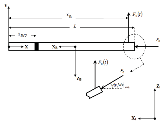
شکل ۱: یک مدل ساده از یک سازه هوافضایی به صورت یک تیر دو سر آزاد به همراه میرایی
