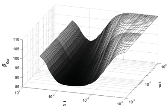
شکل ۵: تاثیر \bar{\alpha} و \bar{\beta} بر مقدار P_{0cr} در حالت \bar{\alpha} \neq 0 و \bar{\beta} \neq 0
