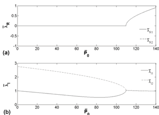
شکل ۴: تغییرات دو مقدار ویژه ابتدایی ماتری اصلی نسبت به تغییرات P_0 ، (الف) بخش حقیقی مقادیر ویژه، (ب) بخش موهومی مقادیر ویژه
