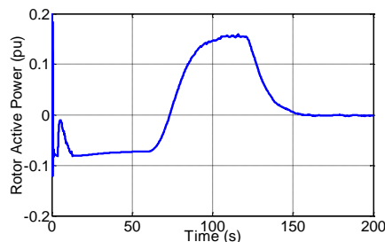
شکل ۱۵ - شکل موج توان اکتیو روتور
