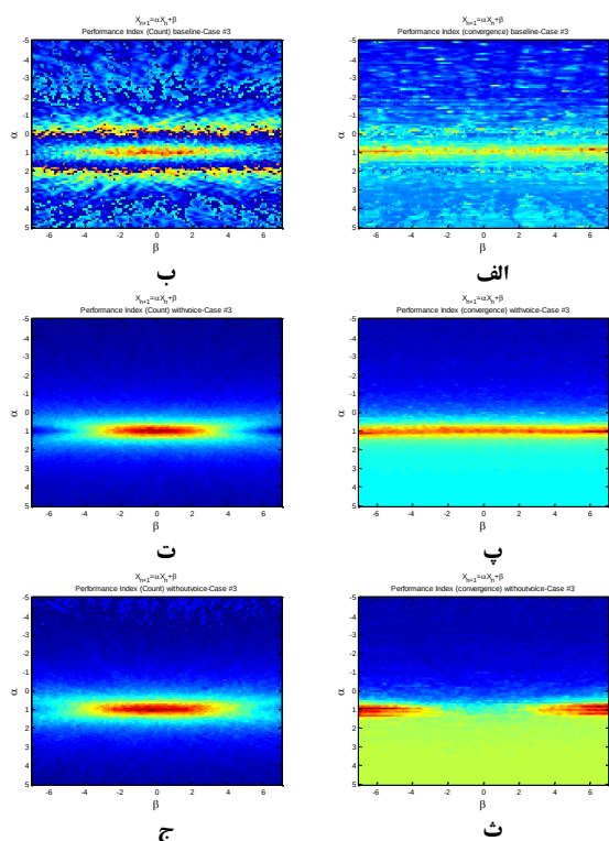
شکل ۹. بررسی صفحه پوانکاره بهینه یک بعدی در اتیسم (فضای بازسازی شده‌ی نسبی تگر) سمت چپ معیار بیشترین تعداد برخورد، سمت راست معیار بیشترین بسط سیگنال
