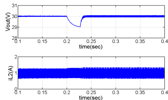
شکل ۱۳: ولتاژ خروجی v_{out} و جریان ورودی i_{L2} وقتی بار خروجی از ۱.۲A به ۲.۴A تغییر می‌کند.
