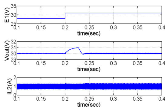
شکل ۱۱: ولتاژ خروجی v_{out} و جریان ورودی i_{L2} وقتی E_1 تغییر می‌کند.
