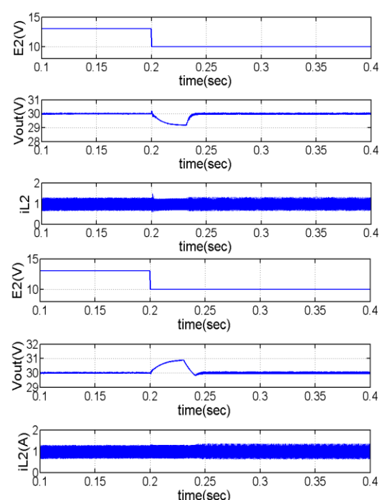
شکل ۱۲: ولتاژ خروجی v_{out} و جریان ورودی i_{L2} وقتی E_2 تغییر می‌کند.
