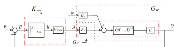
شکل ۴: سیستم کنترل غیر متمرکز برای کنترل مبدل سپیک دو ورودی
