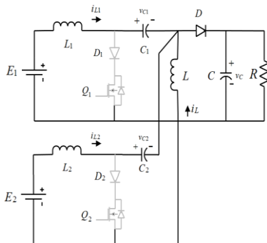
۲- ج حالت عملکردی سوم: Q_1 و Q_2 خاموش
