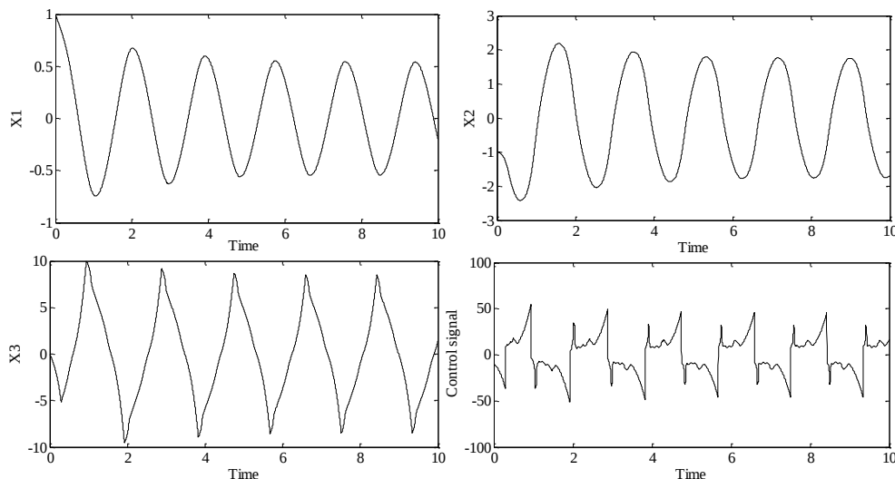
شکل ۶: پاسخ زمانی حالات X_1 ، X_2 و X_3 و سیگنال کنترل u در کنترل مد لغزشی ترمینال (TSM) سیستم کولت در حضور عدم قطعیت و اغتشاش و با ضرایب تصادفی
