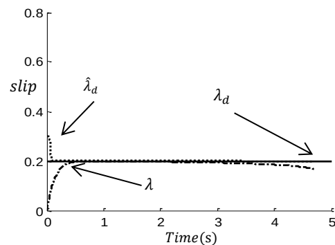
شکل ۱۳: لغزش بهینه تخمین زده شده و لغزش واقعی در جاده نمناک
