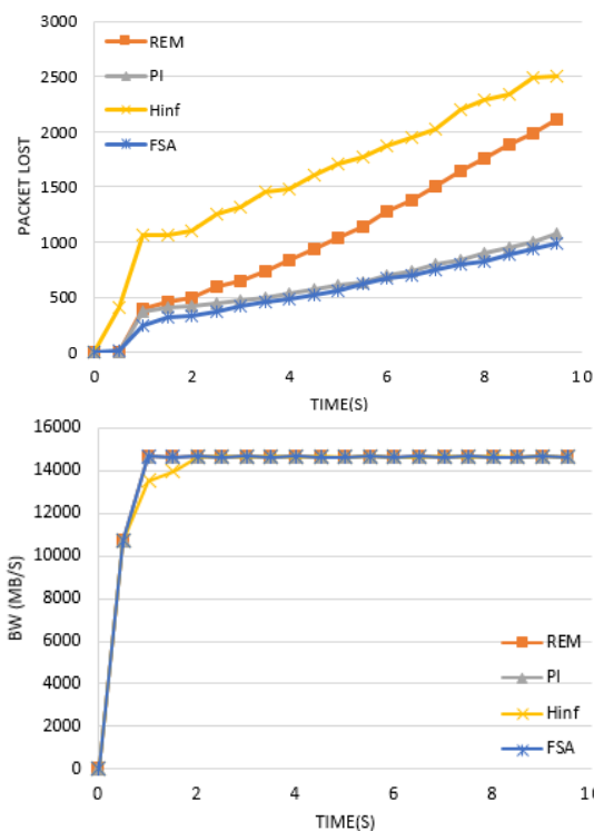
شکل ۵: نمودار حذف بسته در بافر مسیریاب و پهنای باند لینک
