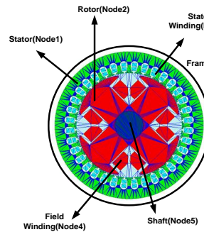
شکل ۴: گره بندی ژنراتور سنکرون به منظور محاسبه خازنهای پارازیتی
