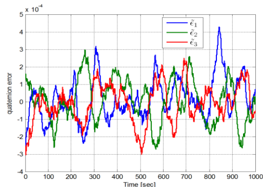
شکل ۱۲: خطای کوآترنیون ردیابی مسیر مطلوب در مود ۳
