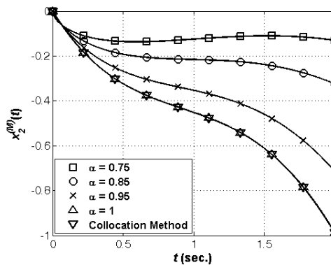
شکل ۵: نمودارهای حالت زیر-بهینه مرتبه پنجم x_2^{(5)}(t) محاسبه شده توسط روش سری مودال به ازای مقادیر مختلف \alpha به همراه روش کولوکیشن (مثال ۲).
