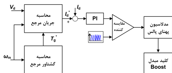
شکل ۱۰: استراتیژی کنترل یکسو ساز و مدل پوست
