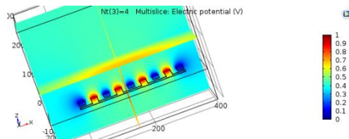
شکل ۲۱: تصویر مربوط توزیع پتانسیل الکتریکی برای تعداد ۴ شانه-نمای ۲
