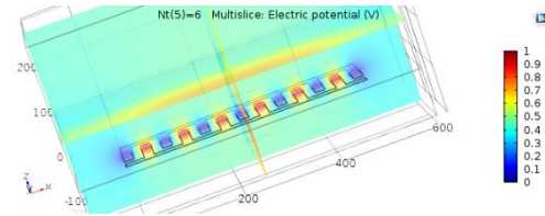
شکل ۲۴: تصویر مربوط توزیع پتانسیل الکتریکی برای تعداد ۶ شانه-نمای ۱
