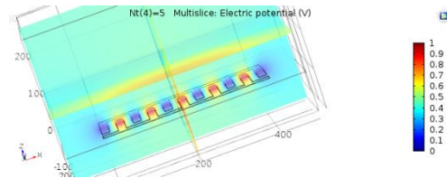
شکل ۲۲: تصویر مربوط توزیع پتانسیل الکتریکی برای تعداد ۵ شانه-نمای ۱
