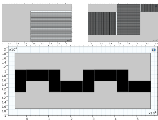
شکل ۵۷: طرح و ماسک مربوط به میکرو کانال تک کانال با الکترودهای شانه ای و منحنی شکل
