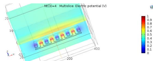
شکل ۲۰: تصویر مربوط توزیع پتانسیل الکتریکی برای تعداد ۴ شانه-نمای ۱
