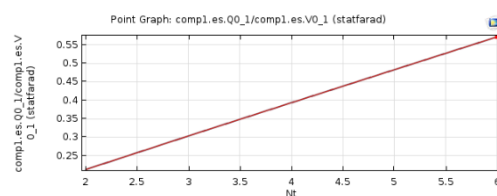
شکل ۳۹: نمودار مربوط به تغییرات میزان خازن شانه ای بر حسب تغییرات تعداد شانه ها
