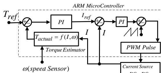
شکل ۱۳: پیاده‌سازی کنترل گشتاور در پردازنده
