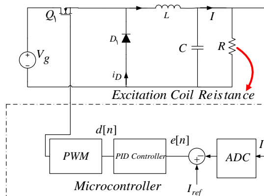
شکل ۸: کنترل جریان مبدل DC-DC
