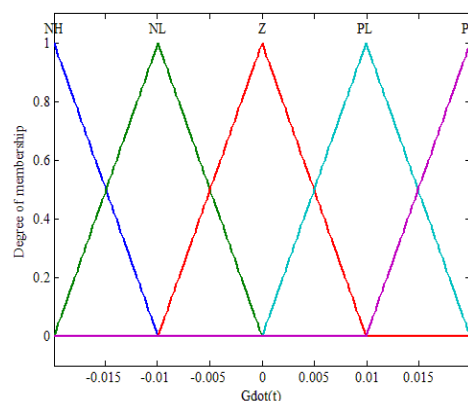
شکل ۶: توابع عضویت ورودی نرخ تغییرات گلوکز \dot{G}(t) با اعمال الگوریتم ژنتیک برای بیمار ۱
