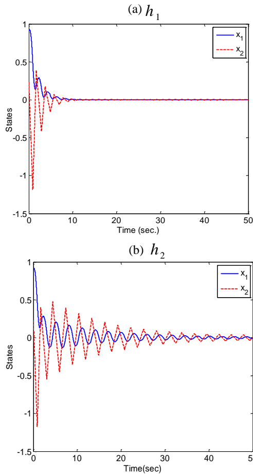
شکل ۴: پاسخ زمانی سیستم کنترل
