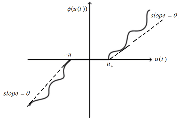
شکل ۲: تابع غیرخطی ناحیه مرده [۳۳].
