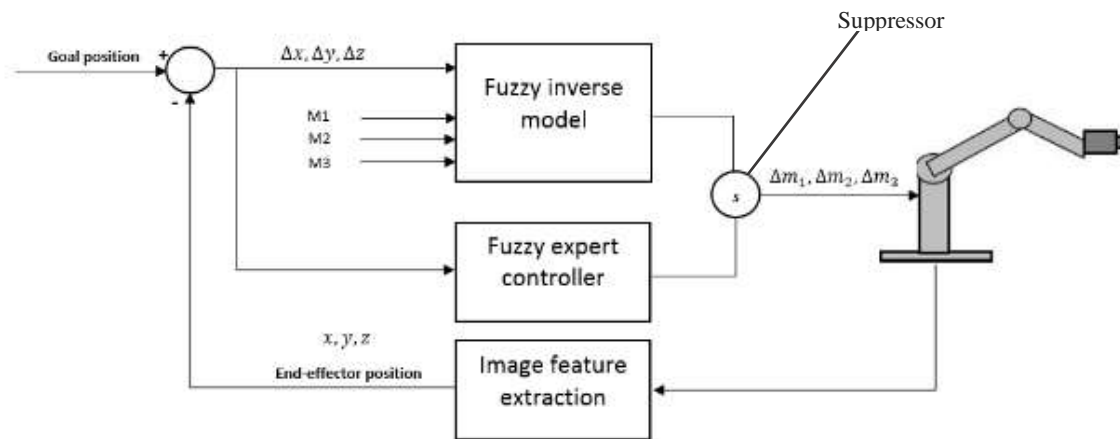
شکل ۵: کنترل گر ترکیبی فازی
