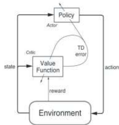
شکل ۳: معماری عملگر-نقاد [۱۳]
