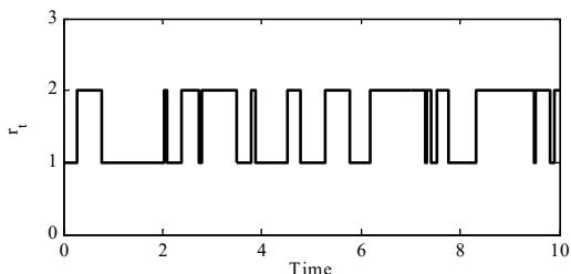
شکل ۲: تغییرات بین دو وضعیت از زنجیره مارکوف سیستم (sigma_t)
