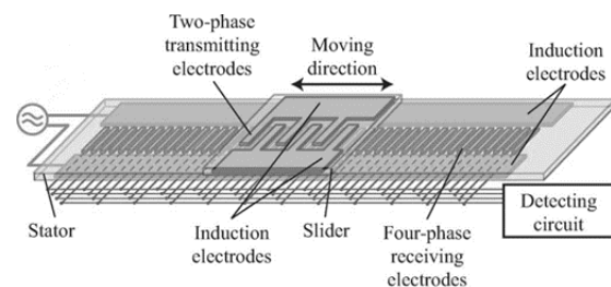
شکل ۳: ساختار شماتیک انکودر خطی با القای الکترواستاتیک خازنی [۷]
