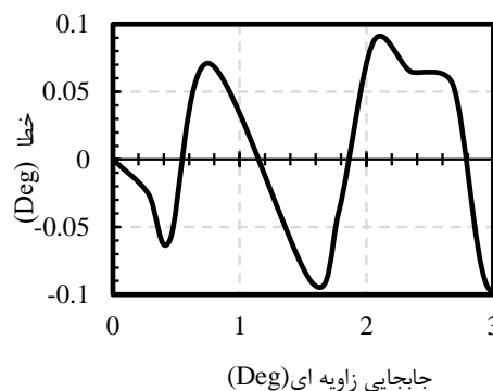
شکل ۱۰: نمودار خطا خروجی انکودر به ازای ۱۰ و ۳ درجه جابجایی
