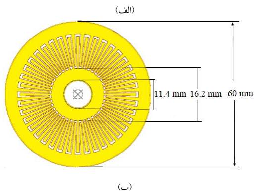
شکل ۵: (الف) نمونه ساخته شده و (ب) مشخصات هندسی روتور انکودر
