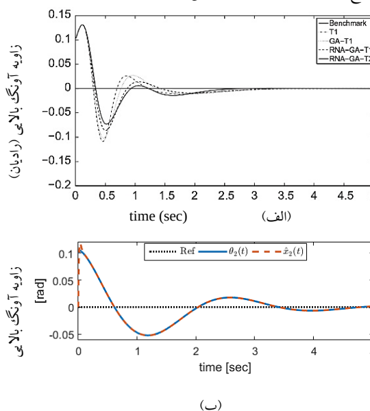
شکل ۱۳: مقایسه نتایج شبیه‌سازی برای زاویه آونگ بالایی. (الف) نتایج مقاله با مقایسه روش‌های مختلف ذکر شده در متن مقاله (ب) نتایج این پژوهش در شکل ۱۴ مقایسه‌ی بین زاویه آونگ پایینی در هر دو حالت مدل این پژوهش و مرجع اشاره شده، ارائه شده است. تفاوت محرز عملکرد دو رویکرد در شروع فرآیند روشن است.
