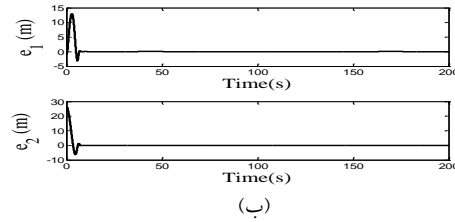
شکل ۱۳- خطاهای ردیابی e_1 و e_2 : (الف) کنترل کننده پیشنهادی (ب) کنترل کننده (۵۵)
