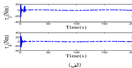
شکل ۱۵- ورودی های کنترل کننده اعمال شده به بدنه متحرک: (الف) کنترل کننده پیشنهادی (ب) کنترل کننده (۵۵)
