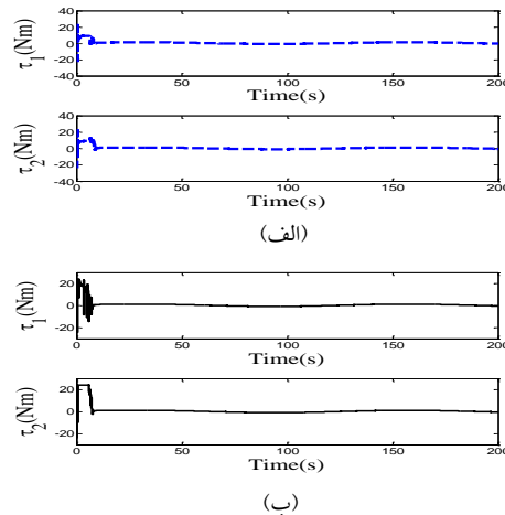
شکل ۱۵- ورودی های کنترل کننده اعمال شده به بدنه متحرک: (الف) کنترل کننده پیشنهادی (ب) کنترل کننده (۵۵)
