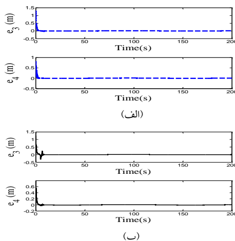
شکل ۱۴- خطاهای ردیابی e_3 و e_4 : (الف) کنترل کننده پیشنهادی (ب) کنترل کننده (۵۵)
