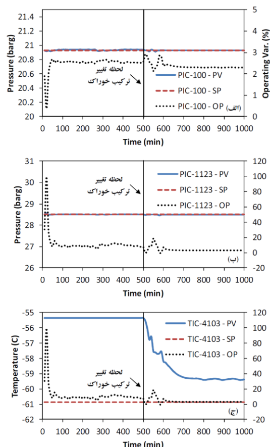
شکل ۱۰: تغییرات مرتبط با کنترل کننده‌های اصلی در شدت جریان خوراک واقعی با استفاده از ضرائب تنظیم ATV: الف) فشار خروجی اکسپندر (PIC-100)، ب) فشار برج اتان زدا (PIC-1123)، ج) دمای خوراک ورودی به برج متان زدا (TIC-4103).
