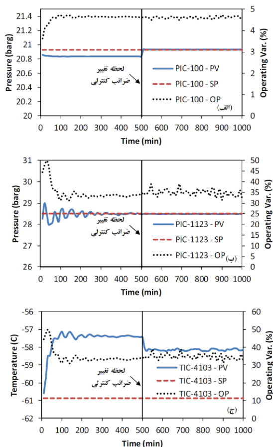
شکل ۶: تغییرات مرتبط با کنترل کننده‌های اصلی در حالت خوراک طراحی:
