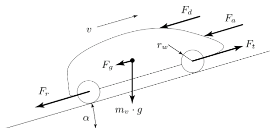
شکل ۲: نیروهای وارده بر خودرو در دینامیک طولی [۱]
