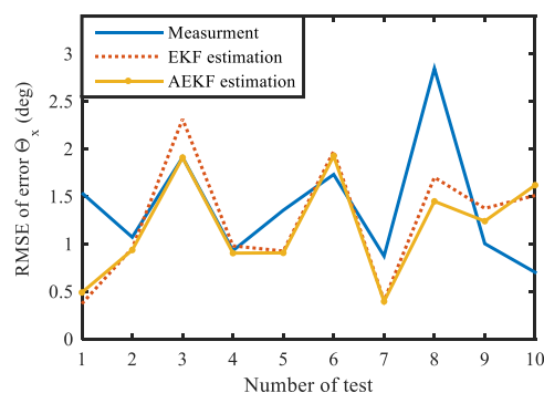
شکل ۲۰: RMSE خطای زاویه برای ۱۰ نمونه داده در سناریوی سرعت متغیر، حالت ناهم‌زمان
