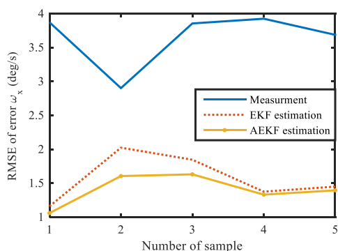
شکل ۱۷: RMSE خطای زاویه‌ای برای ۱۰ نمونه داده در سناریوی سرعت ثابت، حالت هم‌زمان
