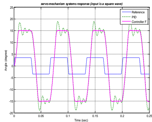
شکل ۱۱: نمودار خروجی به ازای یک ورودی مربعی
