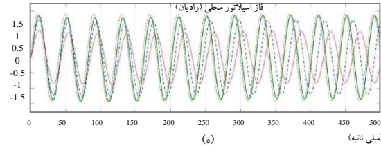
پاسخ سیستم پیشنهادی به تحریک اعمال شده پاسخ PLL با سیستم فازی نوع اول [۴۲،۴۳] پاسخ PLL مرتبه دوم معمولی [۴۰،۴۲]
