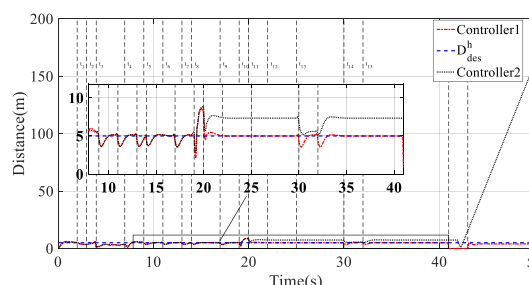
شکل ۱۳: فاصله بین هگزاروتور و هدف زمینی متحرک
