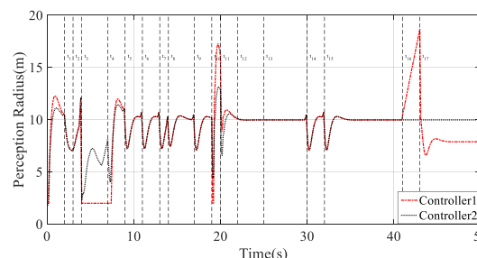
شکل ۱۲: شعاع دید هگزاروتور
