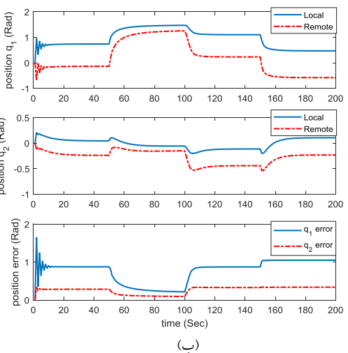
شکل ۶: موقعیت و خطای ردیابی موقعیت در سیستم عمل از دور کنترل شونده با (T) با روش موردنظر (ب) با روش مقاله [۲۰] در فضای مفصلی.
