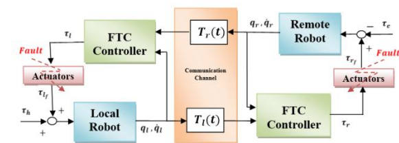
شکل ۲: سیستم عمل از دور دوطرفه مورد نظر
