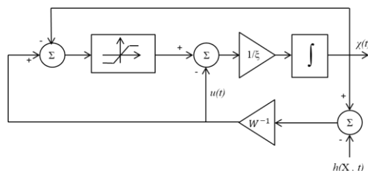
شکل ۳: نمودار بلوکی شبکه عصبی بازگشتی مبتنی بر نظریه تصویر برای حل
