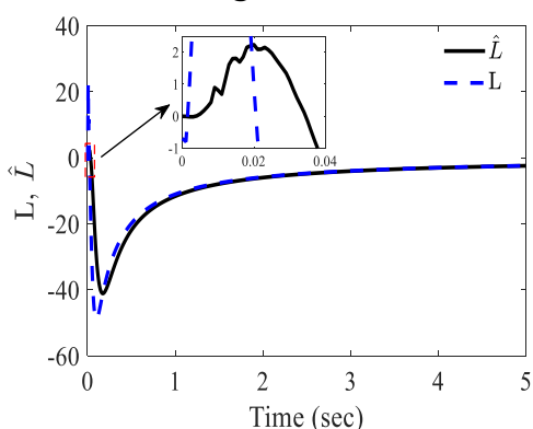
شکل ۶-د: مقایسه عملکردهای RBFNN-PbC و PbC در مانور ۱،
