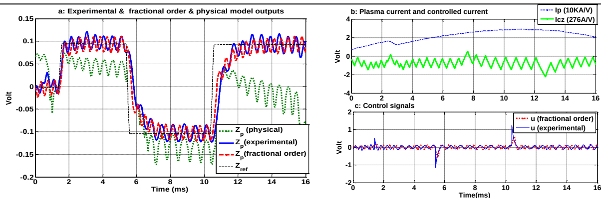
شکل ۱۷: مکان عمودی پلاسما برای شات ۲۲. b- جریان پلاسما ( I_p )، جریان کنترلی I_{cz} ، c- سیگنال کنترلی عملی و حالت شبیه سازی با مدل کسری
