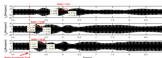
شکل ۱۴- بزرگنمایی شده جریانهای تغذیه موتور القایی در شرایط عیب
