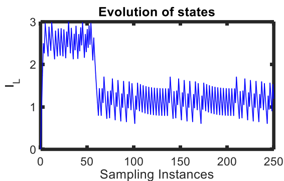
شکل ۹. سیگنال جریان سلف در افق پیش‌بین n_y = 4 .
