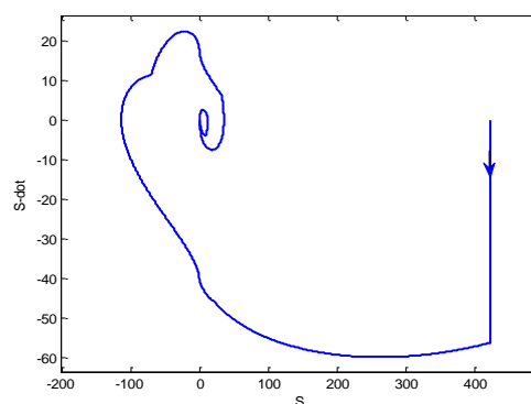
شکل ۱۱: منحنی سطح لغزش بر حسب مشتق اول سطح لغزش برای قانون هدایت پیشنهادی در سناریوی درگیری اول
