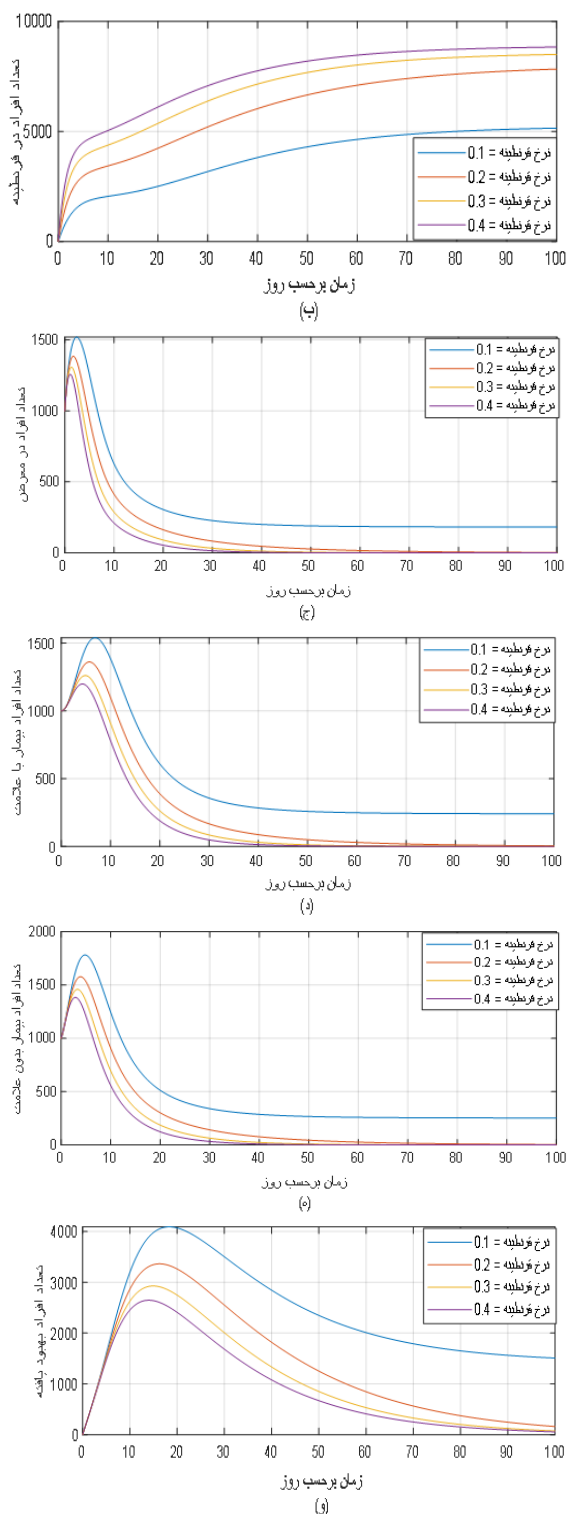
شکل ۲: تأثیر نرخ قرنطینه سازی بر مدل SQUEIAR
