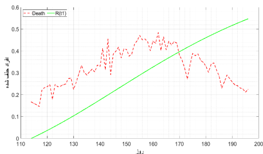
شکل ۳. الف) نمودار مقایسه افراد مبتلا شده در بازه سوم و تخمین مدل از افراد مبتلا (a = 0/063 و b = 0/036) . ب) نقاط قرمز رنگ تعداد افراد فوت‌شده در اثر کرونا و خط سبز رنگ تخمین مدل از افراد حذف‌شده در بازه سوم.
