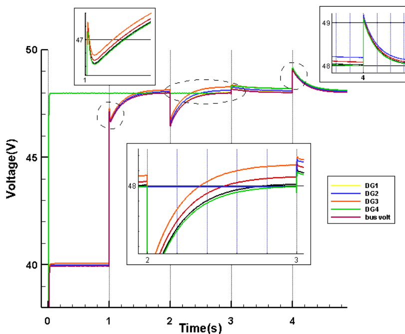
شکل ۱۱: خروجی ولتاژ ریزشیکه DC جزیره‌ای مورد آزمایش در حالت دسترسی همگی DGها به ولتاژ باس اصلی
