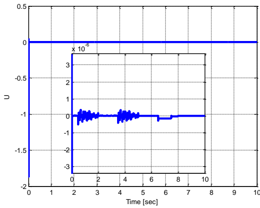
شکل ۹-الف: سیگنال کنترلی
