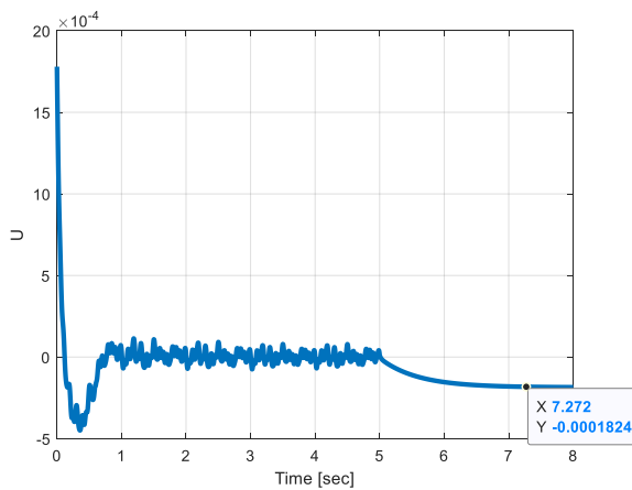
شکل ۵: سیگنال کنترلی
