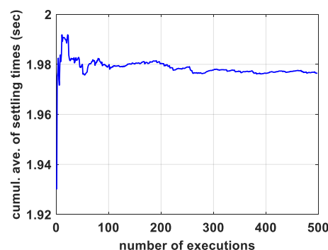
شکل ۲۷: میانگین تجمعی زمان نشست خروجی در ۵۰۰ بار اجرای شبیه‌سازی
