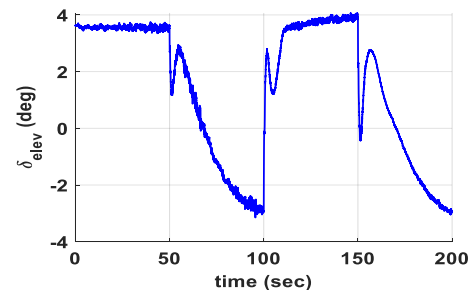
شکل ۲۷: تاریخچه ورودی کنترلی بالابر با حلقه درونی دومرحله‌ای در حضور نویز اندازه‌گیری
