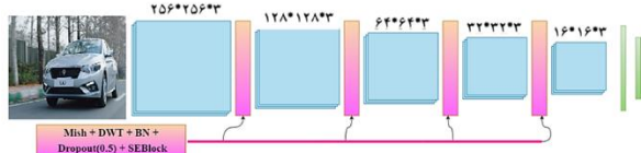
شکل ۱: ساختار طبقه‌بند پیشنهادی
