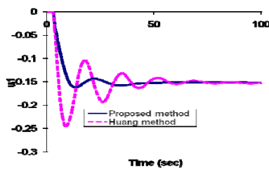
شکل ۱۰. مقایسه پاسخهای خروجی از سیستم کنترل حلقه دوم، به هنگام تغییر پله ای واحد در مقدار مقرر حلقه دوم
