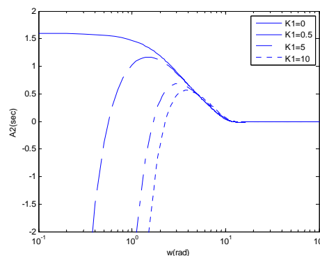
شکل ۱۰: شرط پایداری A_2 به ازای K_2 = 4 ، \alpha = 0 ، \tau_1 = 0.3 ،
