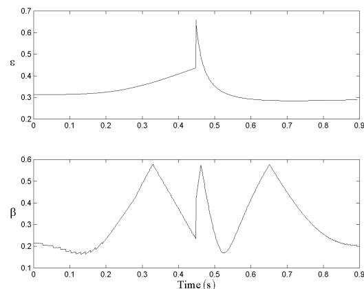
شکل ۱۰- مقادیر متوسط ترک بی‌بعد مفاصل \varepsilon و انحراف ترک‌های بی‌بعد از مقدار متوسط \beta حل بر اساس الگوریتم بهبود ترک
